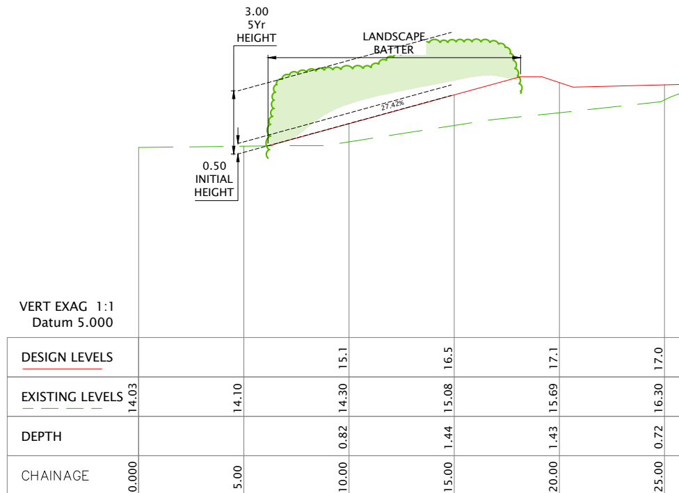
5 SECTION LS01 SCALE: 1:250 @ A3
