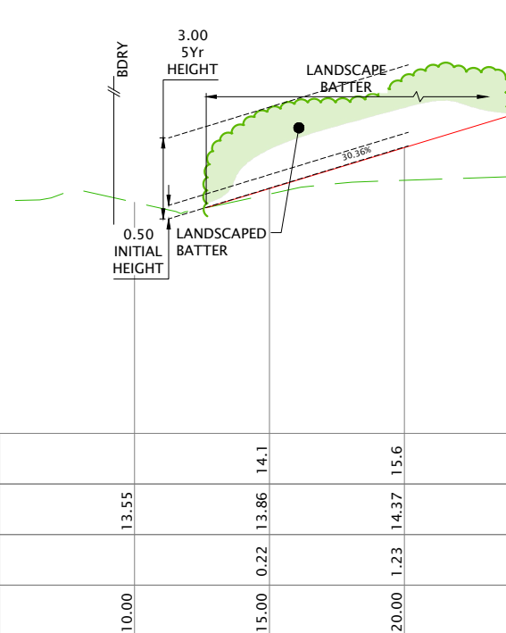
4 SECTION LS01 SCALE: 1:250 @ A3
