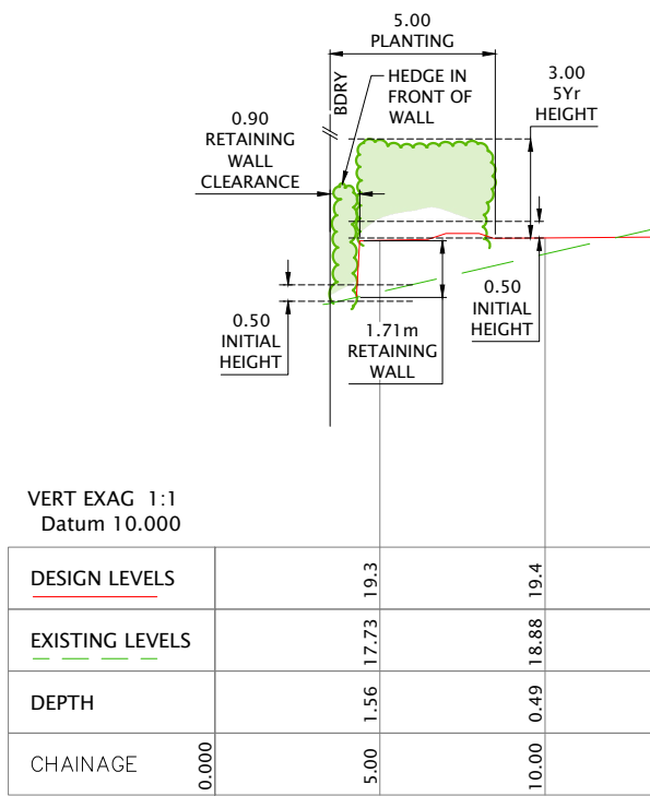
8 SECTION LS01 SCALE: 1:250 @ A3
