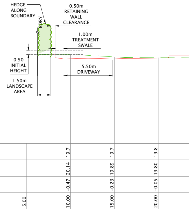
2 SECTION LS01 SCALE: 1:250 @ A3
