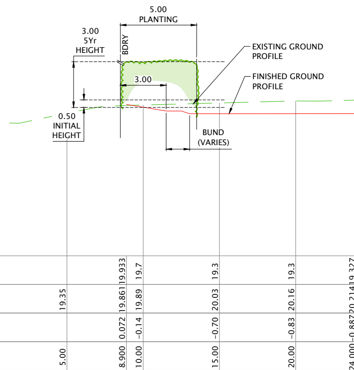
1 SECTION LS01 SCALE: 1:250 @ A3
