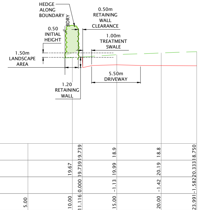
3 SECTION LS01 SCALE: 1:250 @ A3
