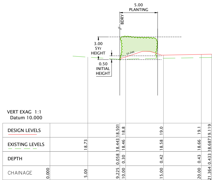
7 SECTION LS01 SCALE: 1:250 @ A3
