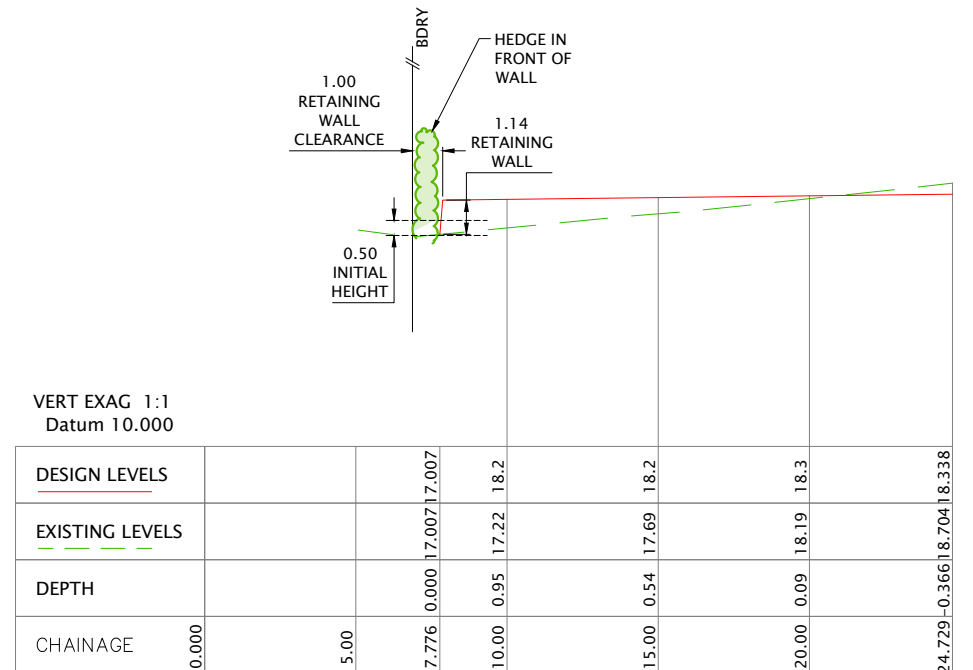
6 SECTION LS01 SCALE: 1:250 @ A3
